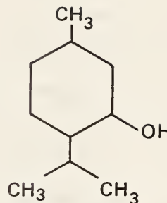
dl - Menthol
